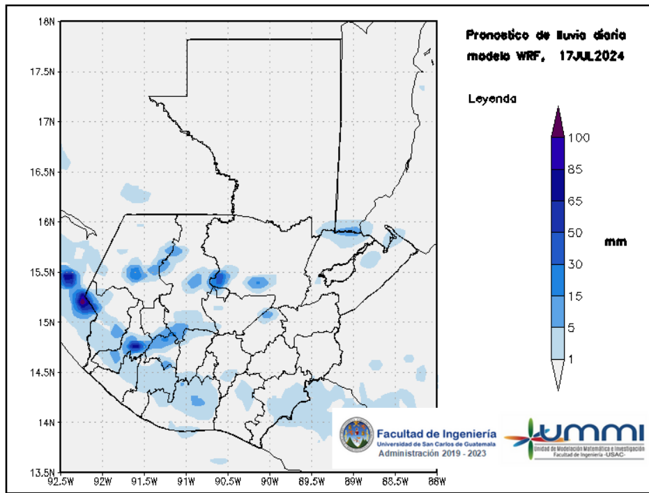
Figura 3: Pronóstico de lluvia diaria del 17 de July
