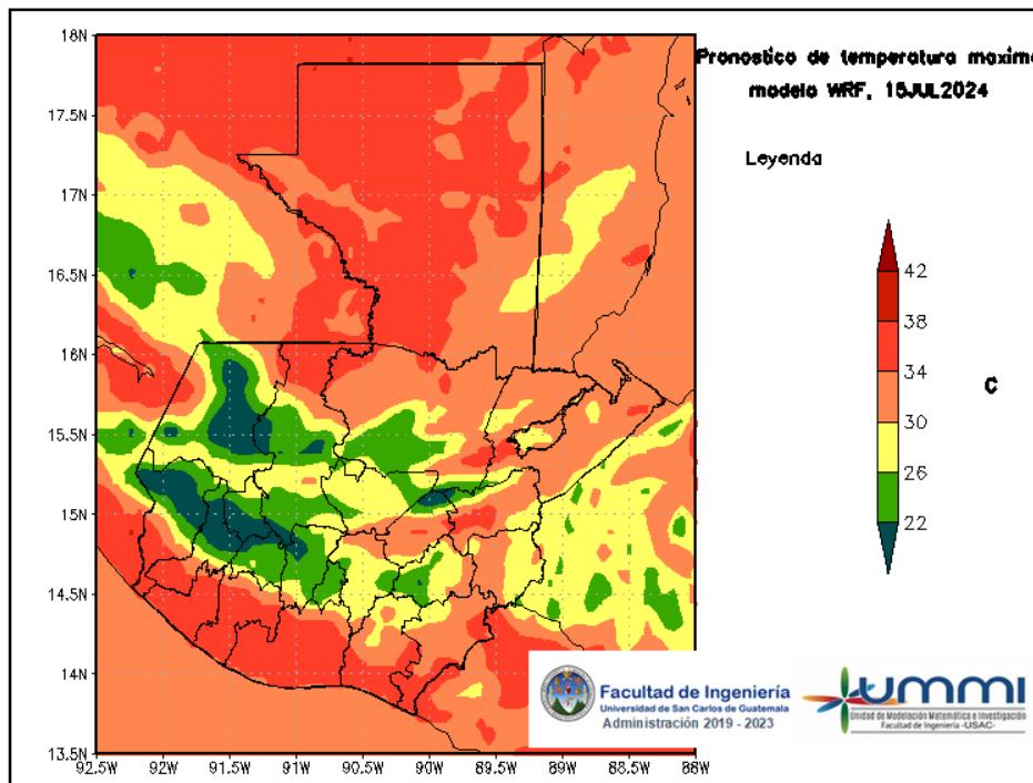
Figura 4: Pronóstico de temperatura máxima diaria del 15 de July
