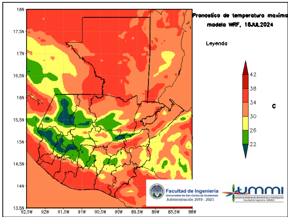
Figura 5: Pronóstico de temperatura máxima diaria del 16 de July
