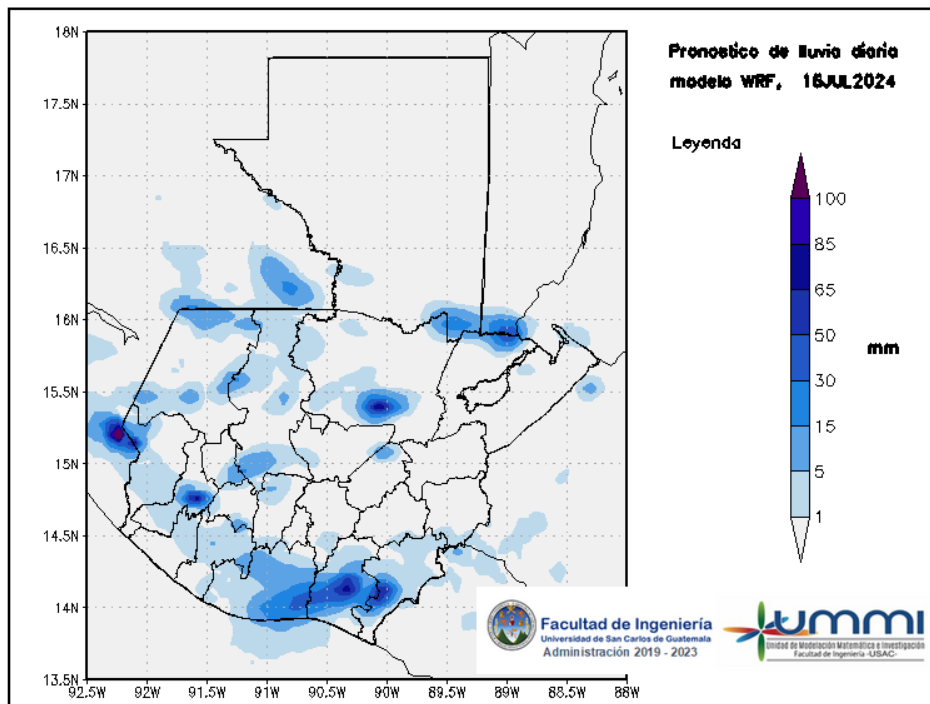
Figura 2: Pronóstico de lluvia diaria del 16 de July
