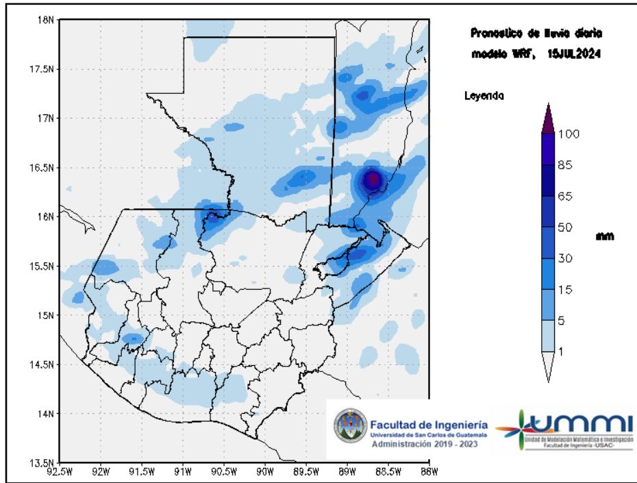
Figura 1: Pronóstico de lluvia diaria del 15 de July
