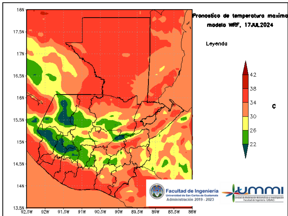
Figura 6: Pronóstico de temperatura máxima diaria del 17 de July
