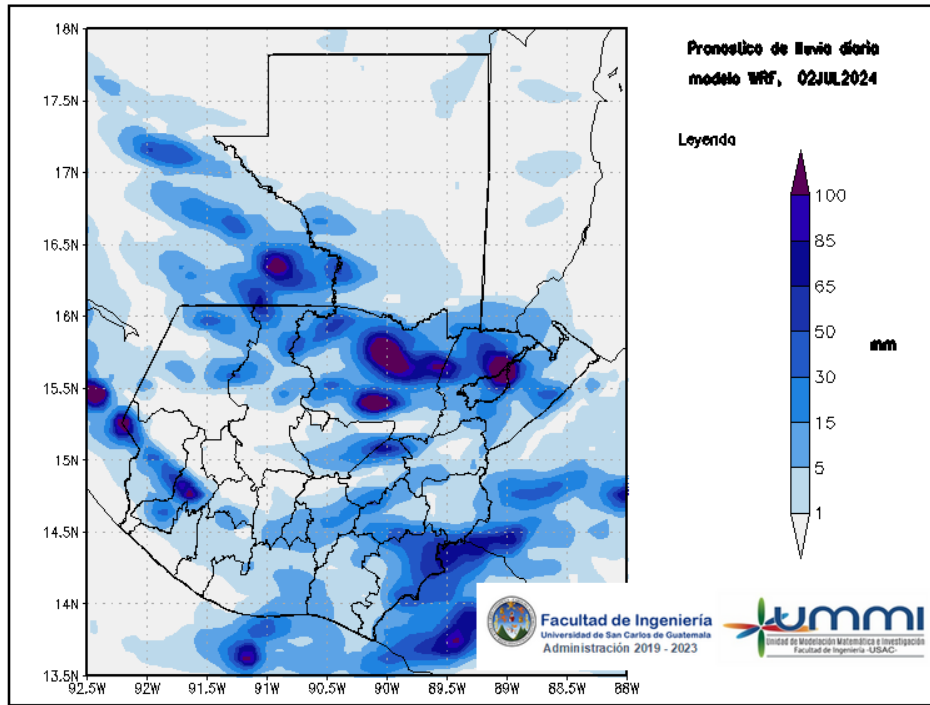
Figura 1: Pronóstico de lluvia diaria del 02 de July
