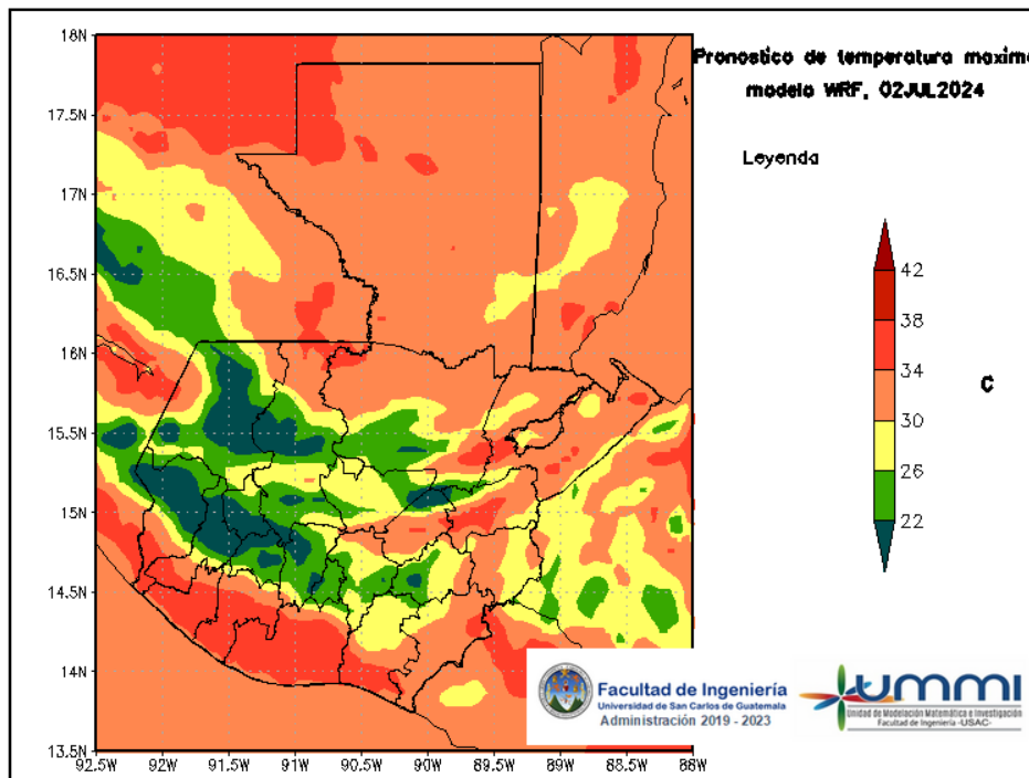
Figura 4: Pronóstico de temperatura máxima diaria del 02 de July
