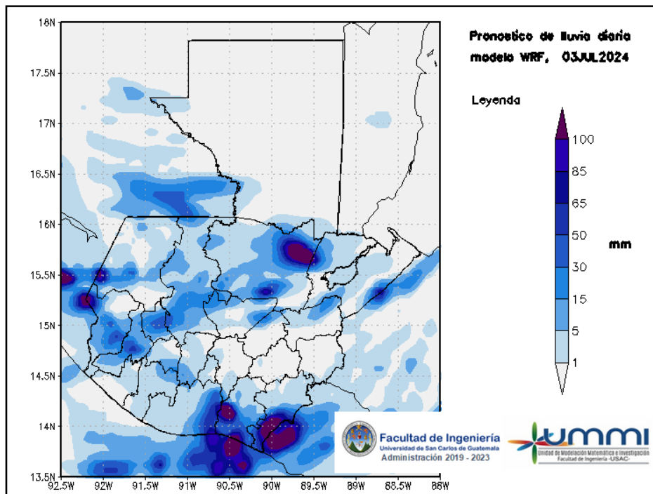
Figura 2: Pronóstico de lluvia diaria del 03 de July
