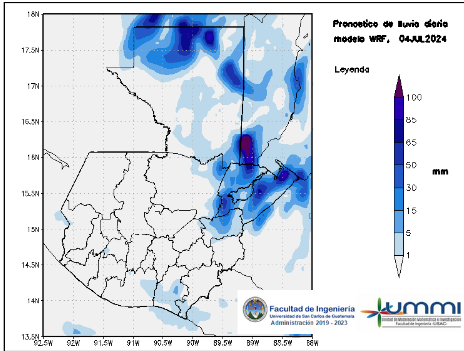
Figura 3: Pronóstico de lluvia diaria del 04 de July
