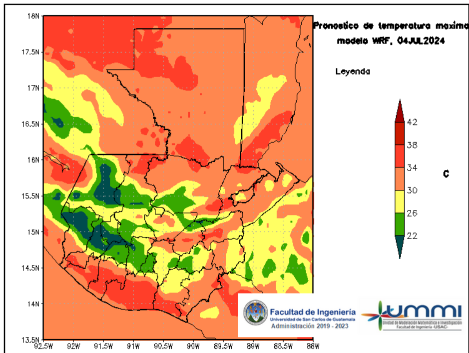
Figura 6: Pronóstico de temperatura máxima diaria del 04 de July
