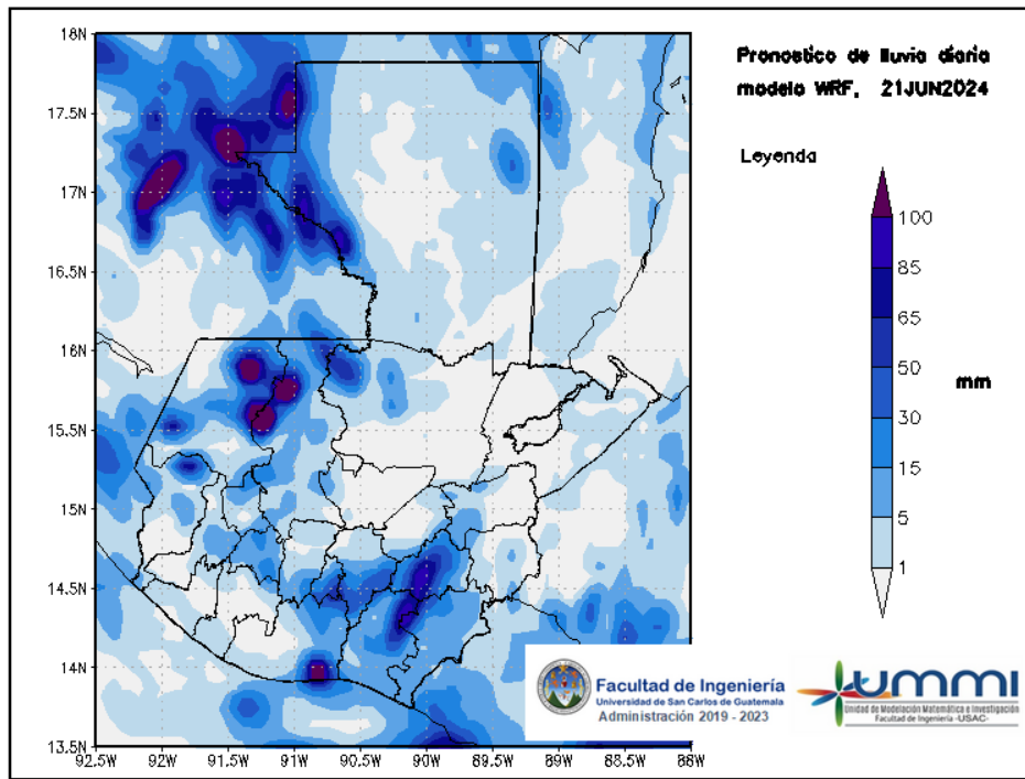
Figura 3: Pronóstico de lluvia diaria del 21 de June
