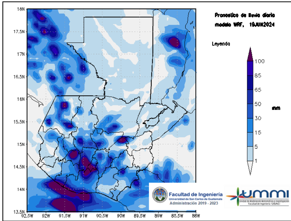
Figura 1: Pronóstico de lluvia diaria del 19 de June
