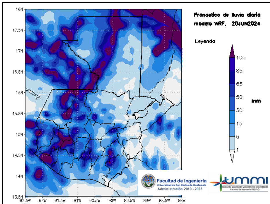
Figura 2: Pronóstico de lluvia diaria del 20 de June
