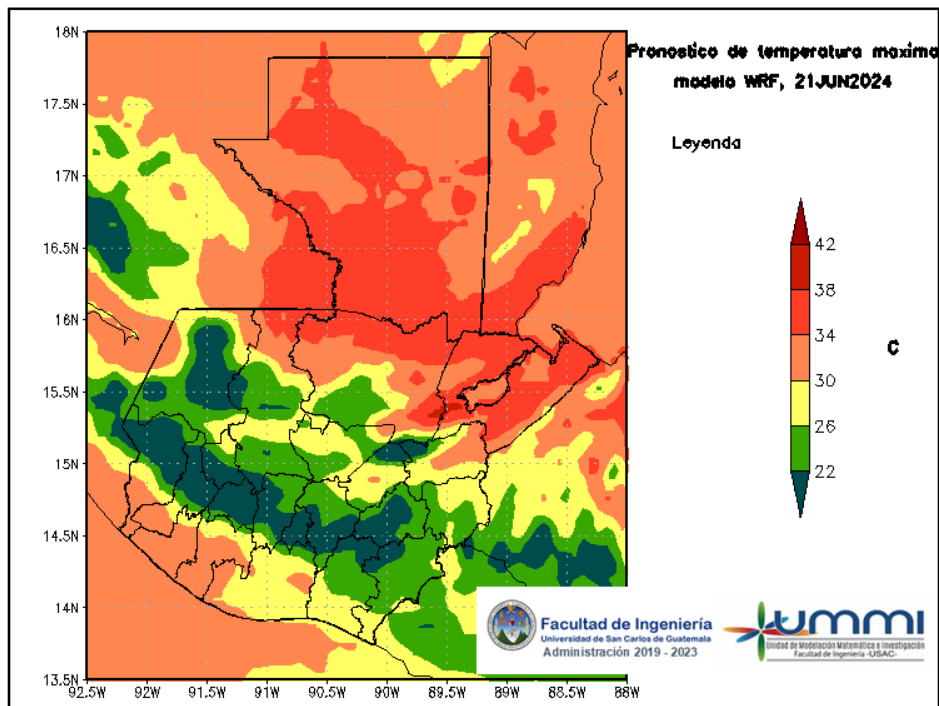
Figura 6: Pronóstico de temperatura máxima diaria del 21 de June
