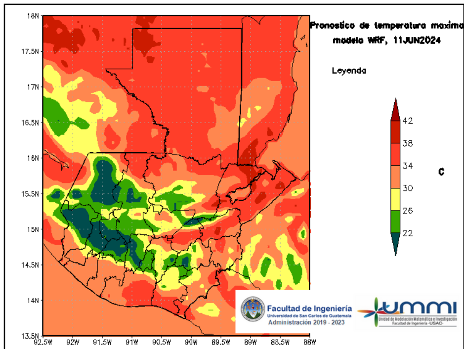
Figura 6: Pronóstico de temperatura máxima diaria del 11 de June
