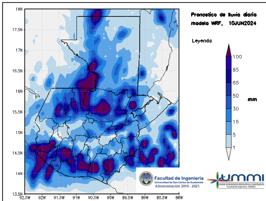
Figura 2: Pronóstico de lluvia diaria del 10 de June
