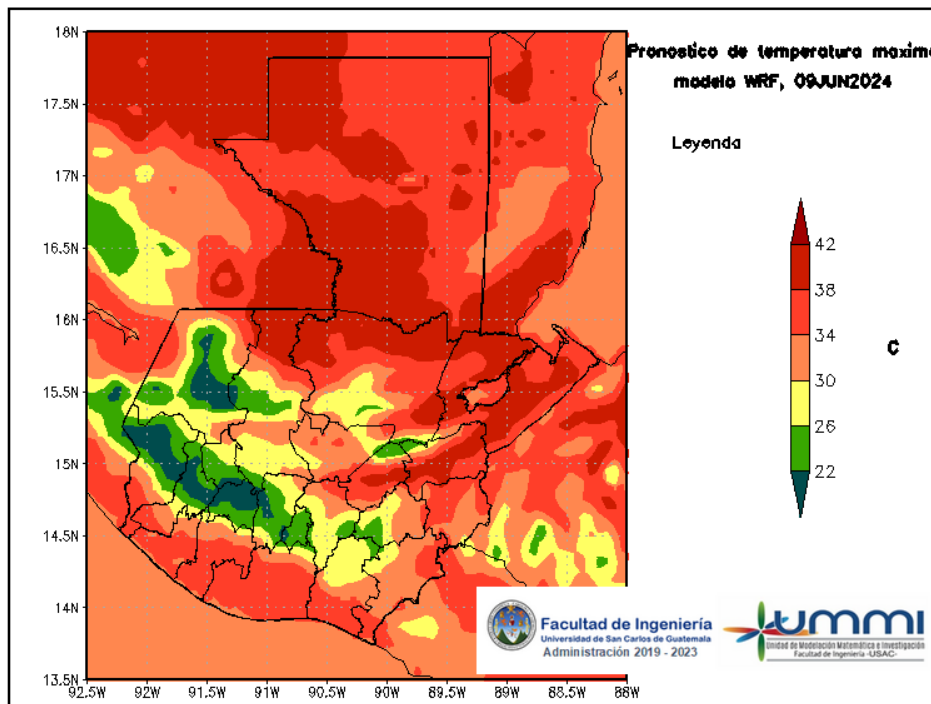
Figura 4: Pronóstico de temperatura máxima diaria del 09 de June
