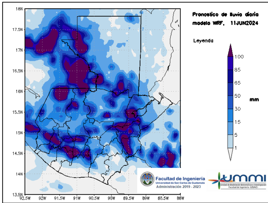
Figura 3: Pronóstico de lluvia diaria del 11 de June
