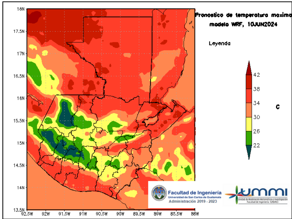
Figura 5: Pronóstico de temperatura máxima diaria del 10 de June
