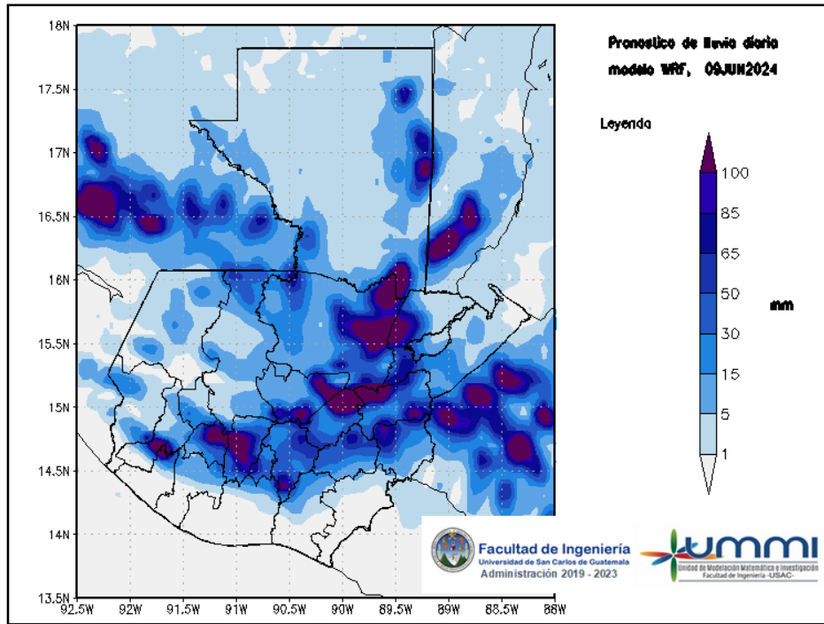
Figura 1: Pronóstico de lluvia diaria del 09 de June
