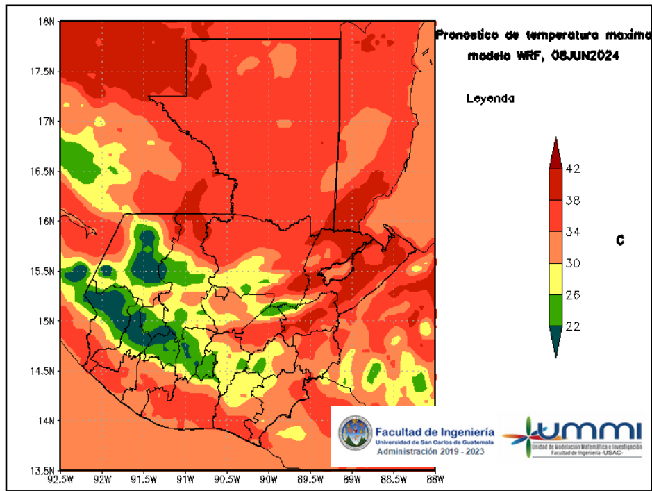
Figura 5: Pronóstico de temperatura máxima diaria del 08 de June
