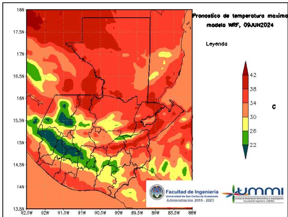
Figura 6: Pronóstico de temperatura máxima diaria del 09 de June
