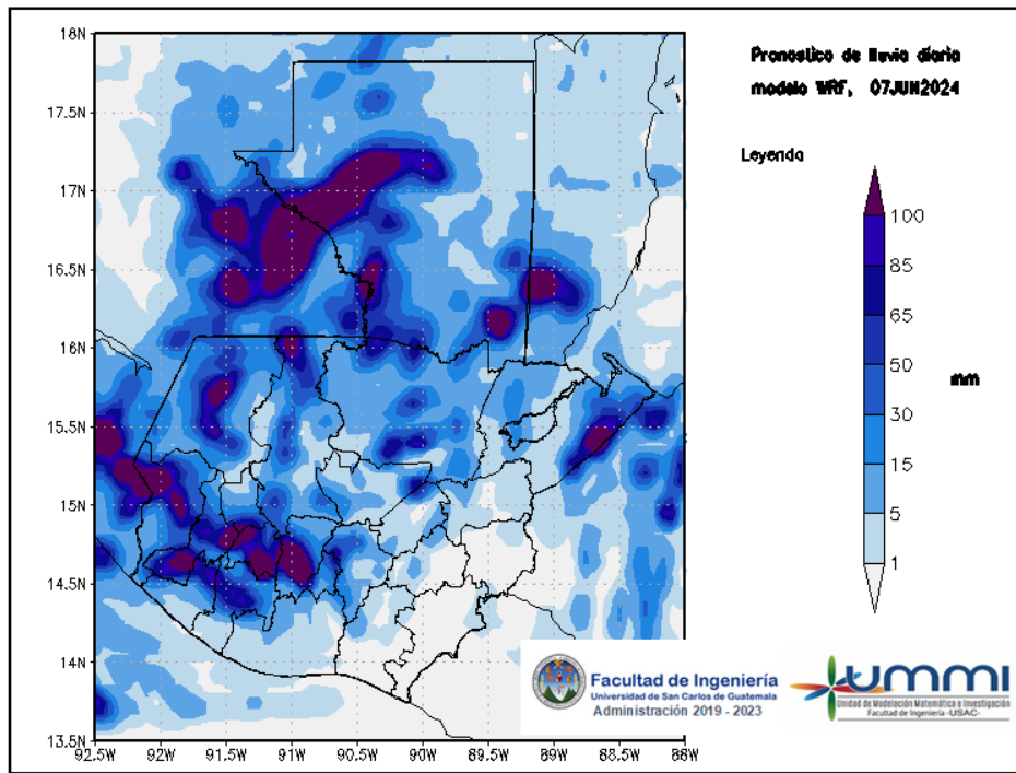
Figura 1: Pronóstico de lluvia diaria del 07 de June
