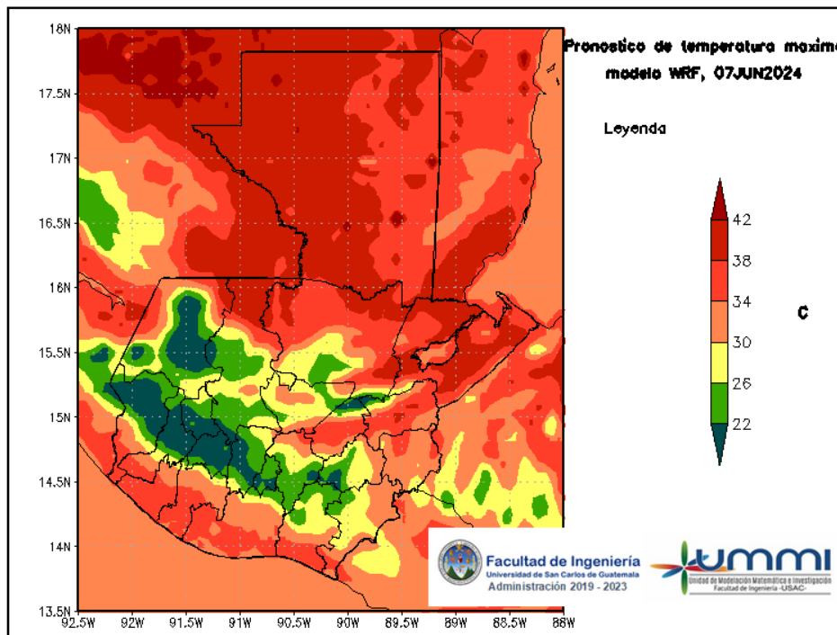
Figura 4: Pronóstico de temperatura máxima diaria del 07 de June
