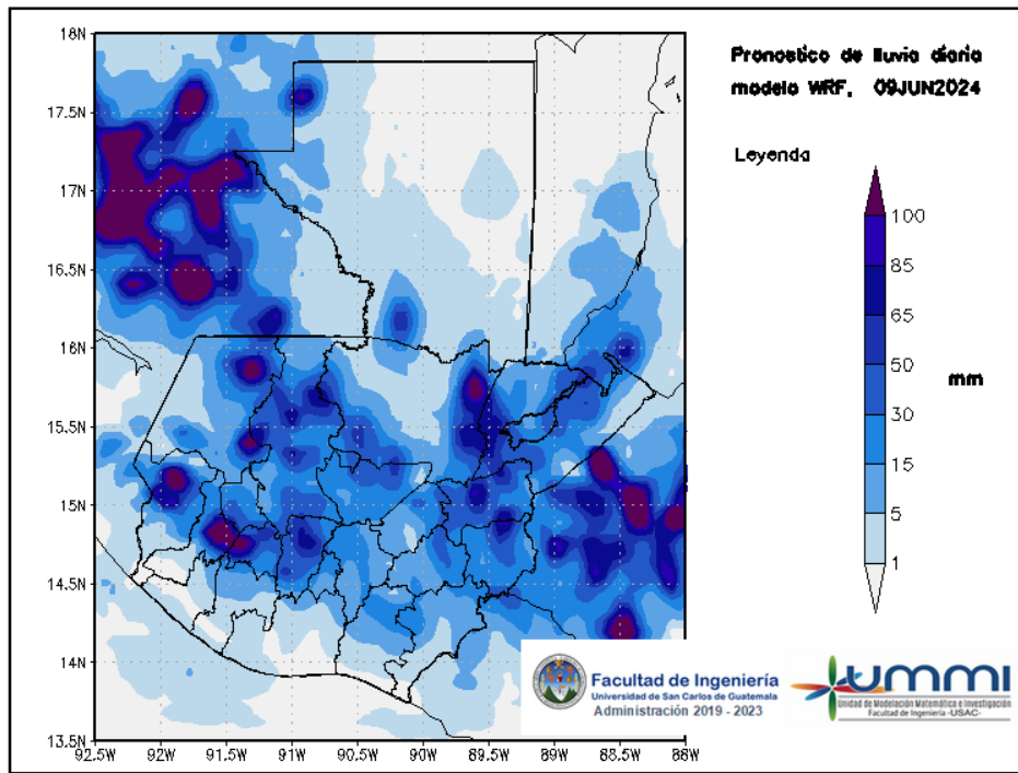
Figura 3: Pronóstico de lluvia diaria del 09 de June
