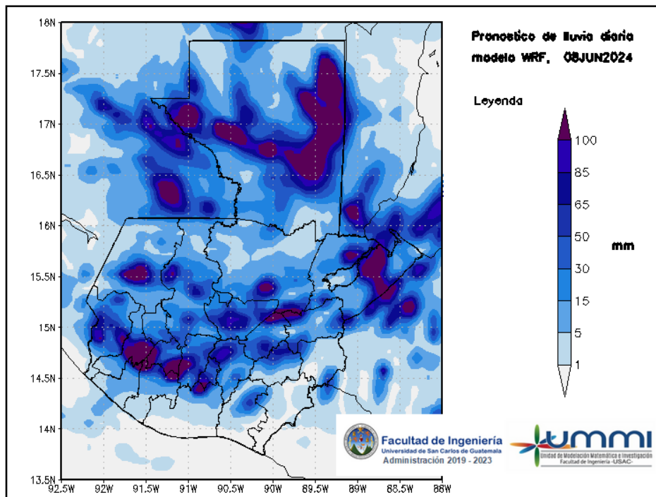
Figura 2: Pronóstico de lluvia diaria del 08 de June
