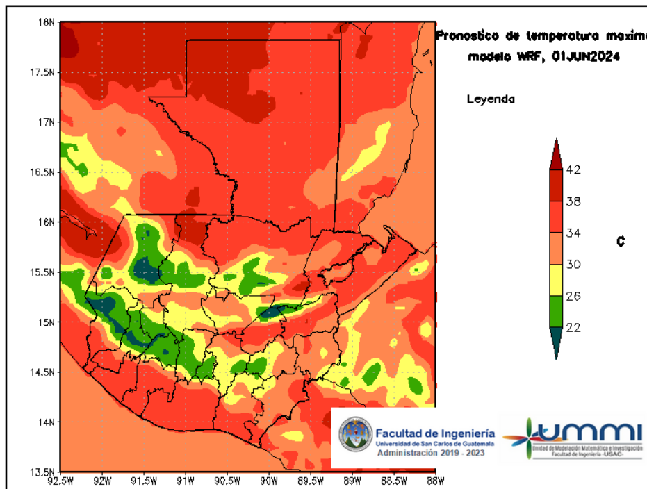
Figura 4: Pronóstico de temperatura máxima diaria del 01 de June
