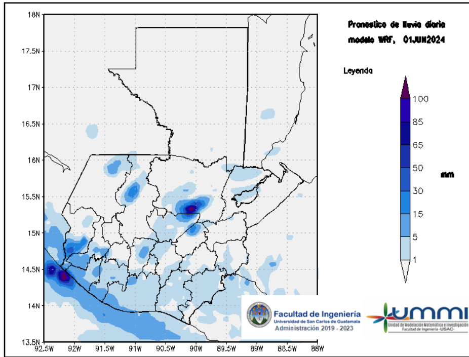
Figura 1: Pronóstico de lluvia diaria del 01 de June
