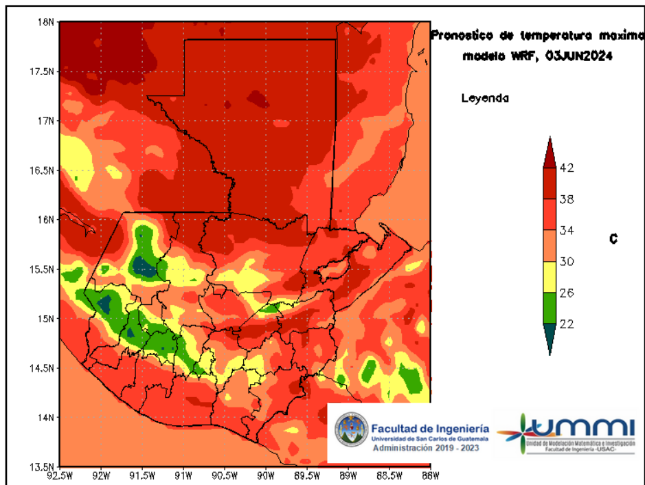
Figura 6: Pronóstico de temperatura máxima diaria del 03 de June
