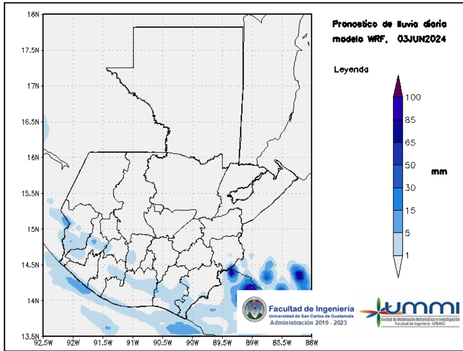
Figura 3: Pronóstico de lluvia diaria del 03 de June
