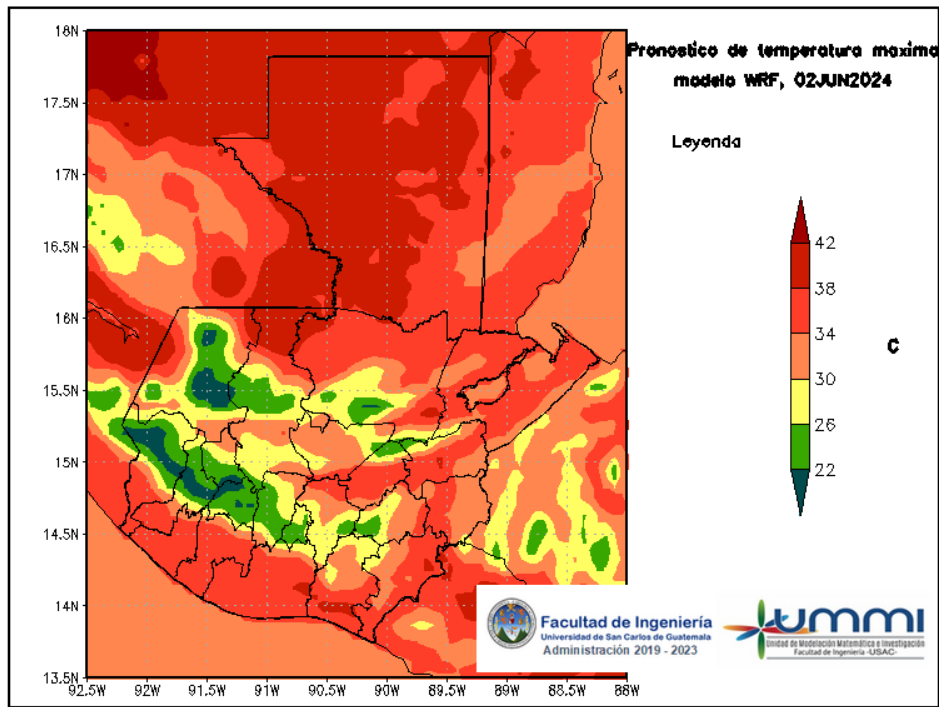
Figura 5: Pronóstico de temperatura máxima diaria del 02 de June
