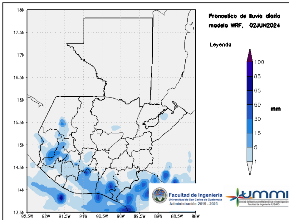
Figura 2: Pronóstico de lluvia diaria del 02 de June
