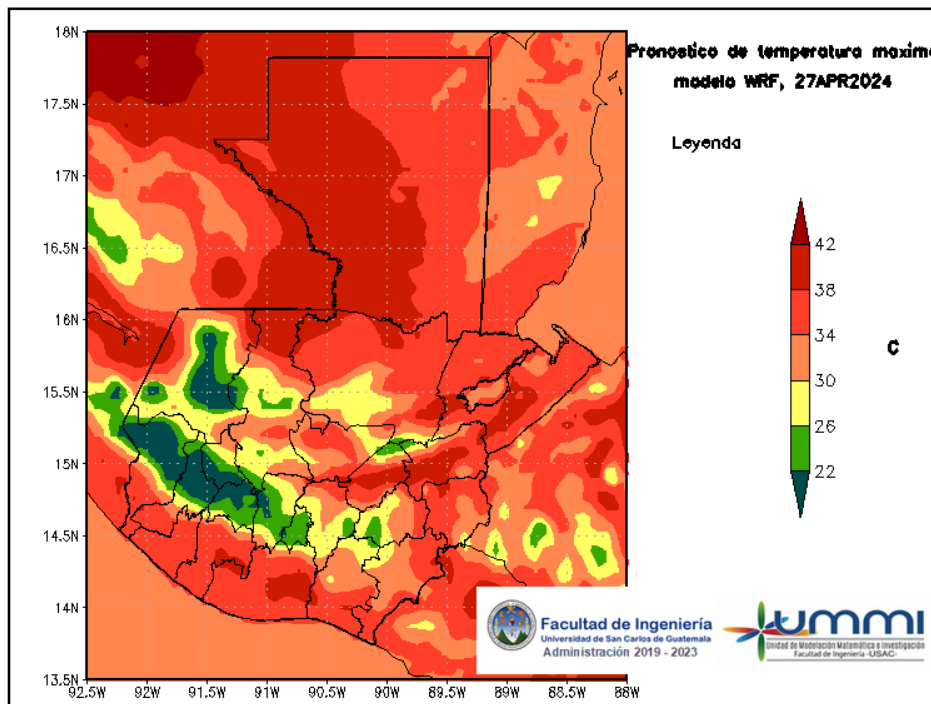
Figura 4: Pronóstico de temperatura máxima diaria del 27 de April
