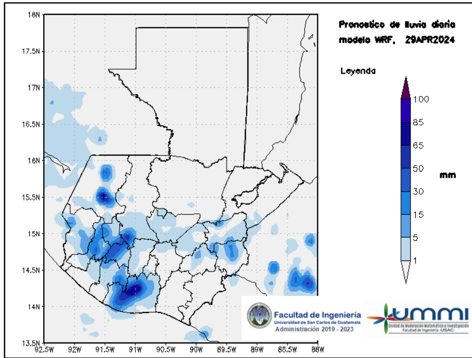
Figura 3: Pronóstico de lluvia diaria del 29 de April
