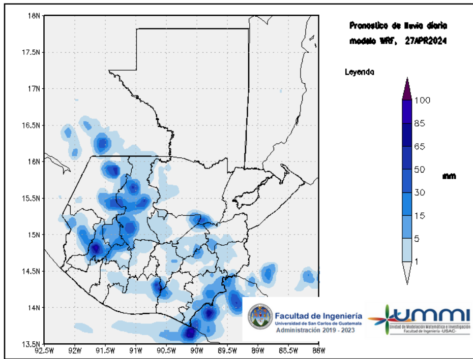
Figura 1: Pronóstico de lluvia diaria del 27 de April
