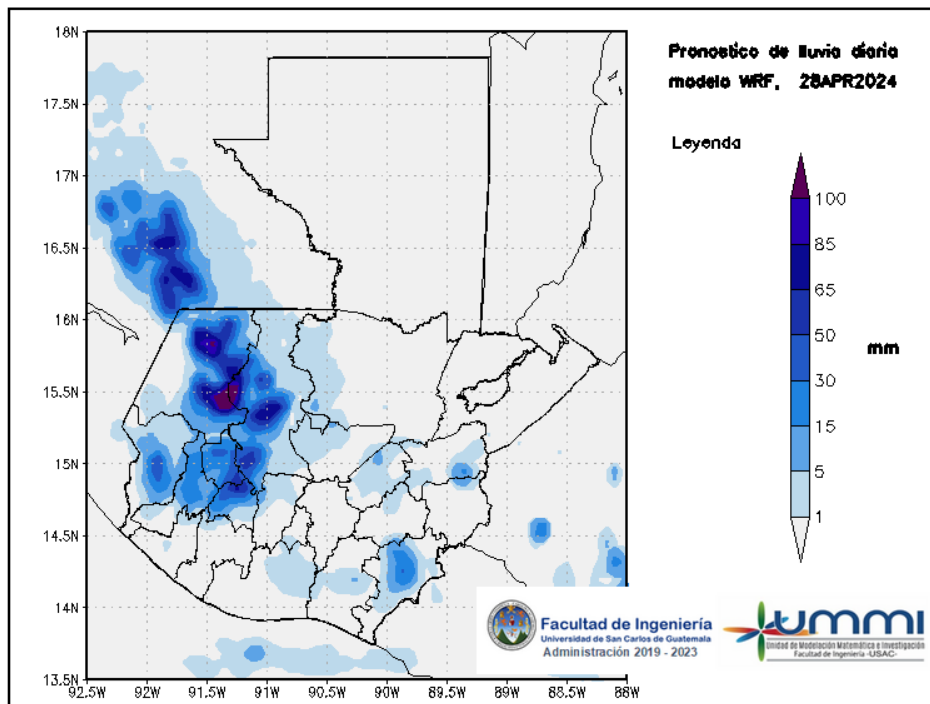
Figura 2: Pronóstico de lluvia diaria del 28 de April
