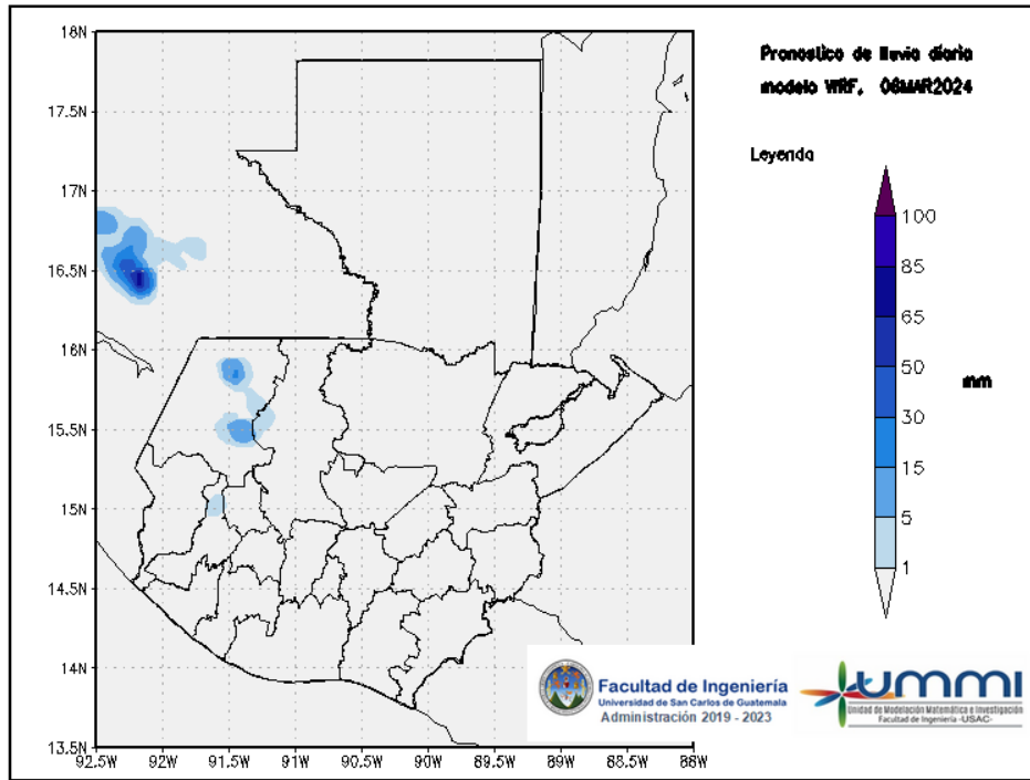
Figura 1: Pronóstico de lluvia diaria del 06 de March
