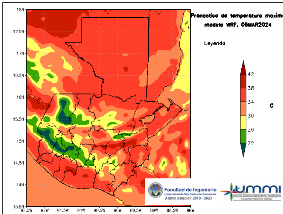
Figura 4: Pronóstico de temperatura máxima diaria del 06 de March
