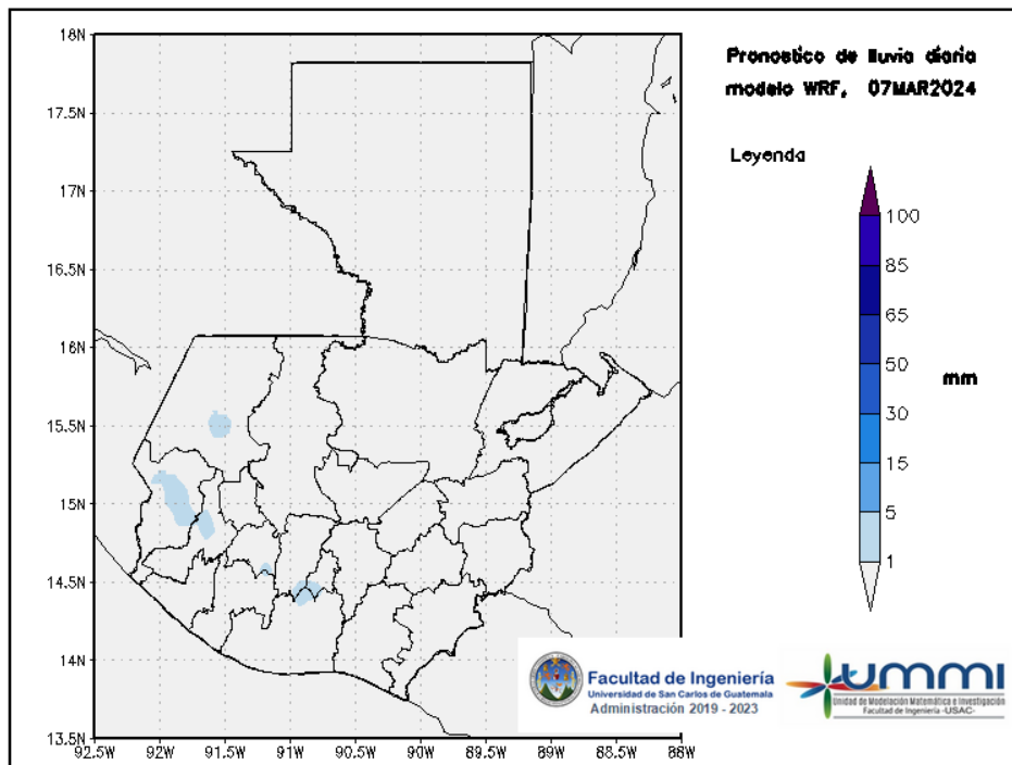
Figura 2: Pronóstico de lluvia diaria del 07 de March
