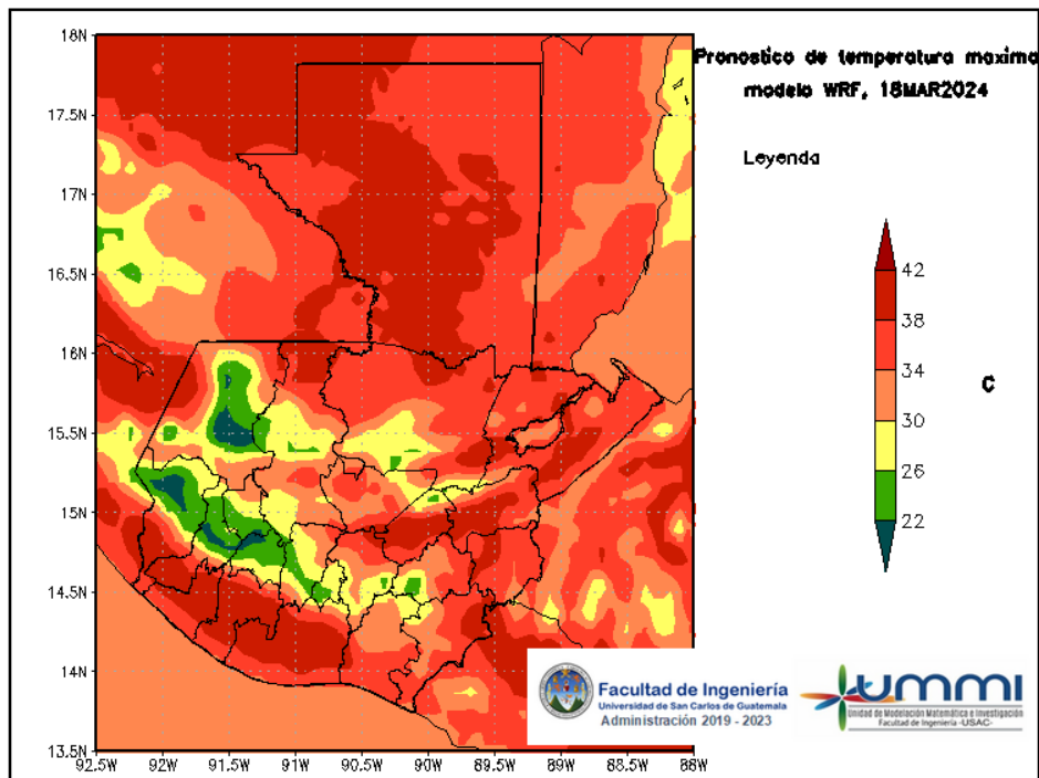
Figura 6: Pronóstico de temperatura máxima diaria del 18 de March
