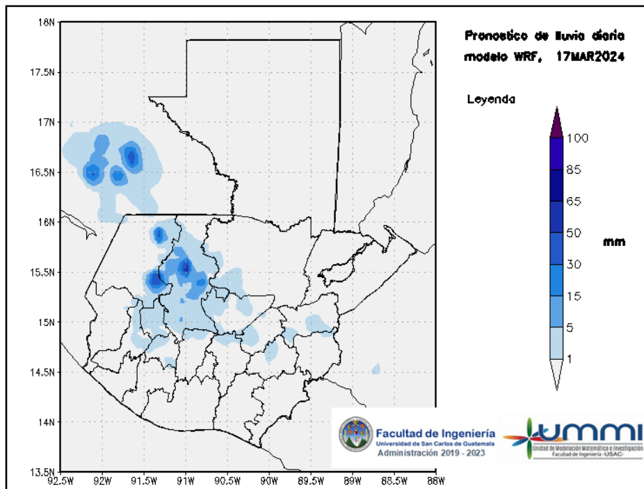
Figura 2: Pronóstico de lluvia diaria del 17 de March
