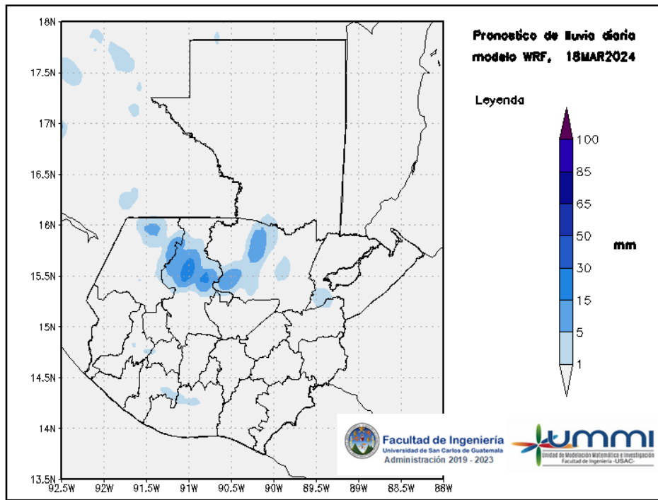
Figura 3: Pronóstico de lluvia diaria del 18 de March
