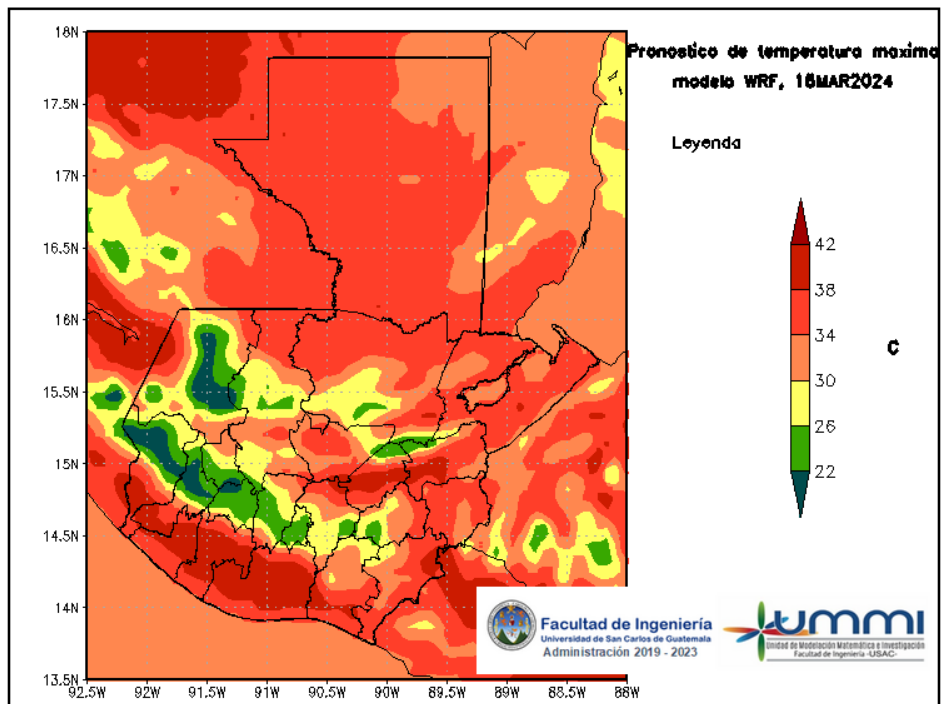
Figura 4: Pronóstico de temperatura máxima diaria del 16 de March
