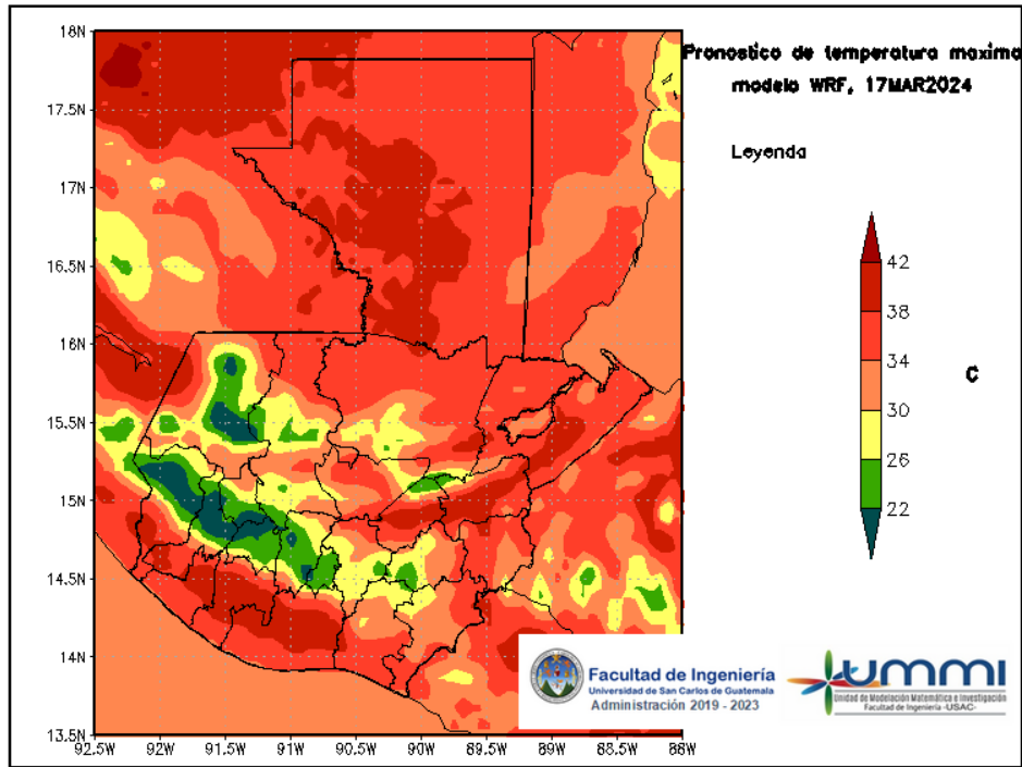
Figura 5: Pronóstico de temperatura máxima diaria del 17 de March
