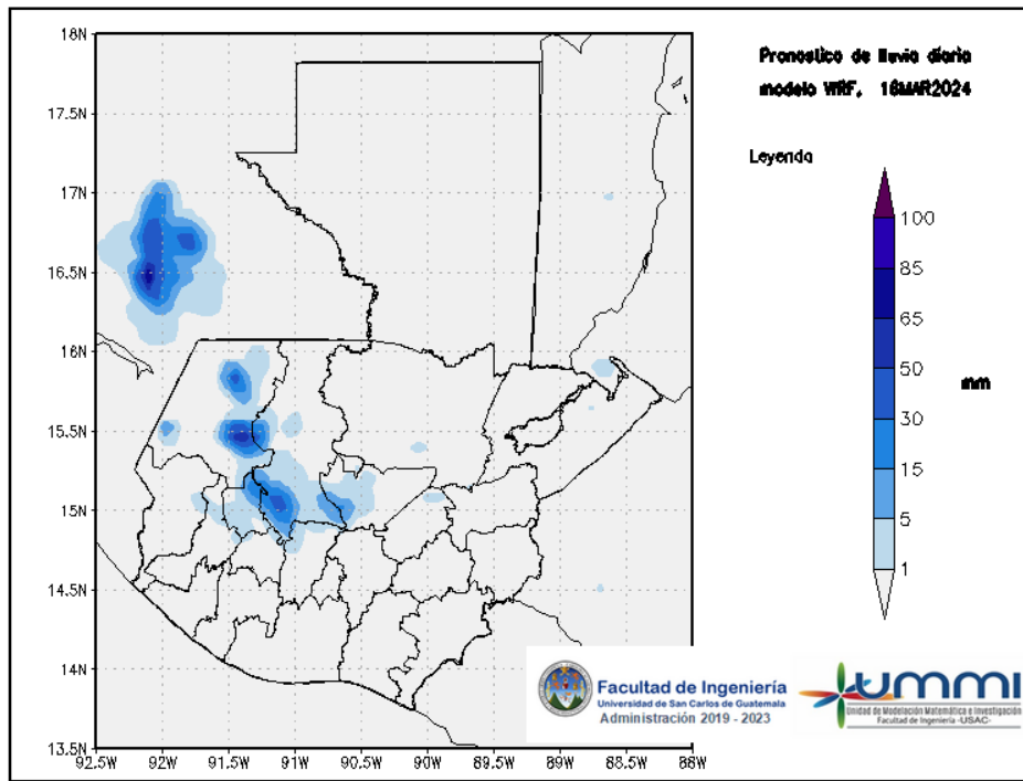
Figura 1: Pronóstico de lluvia diaria del 16 de March
