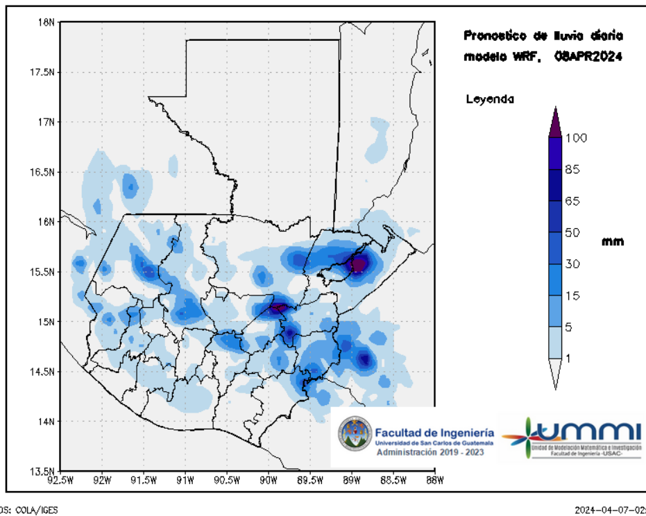
Figura 2: Pronóstico de lluvia diaria del 08 de April
