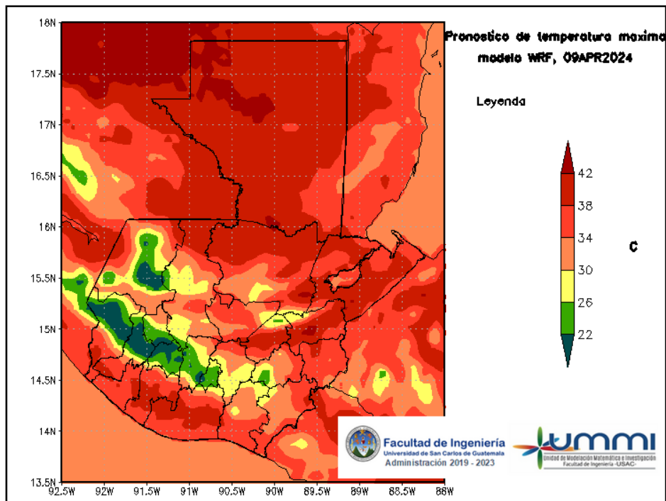
Figura 6: Pronóstico de temperatura máxima diaria del 09 de April
