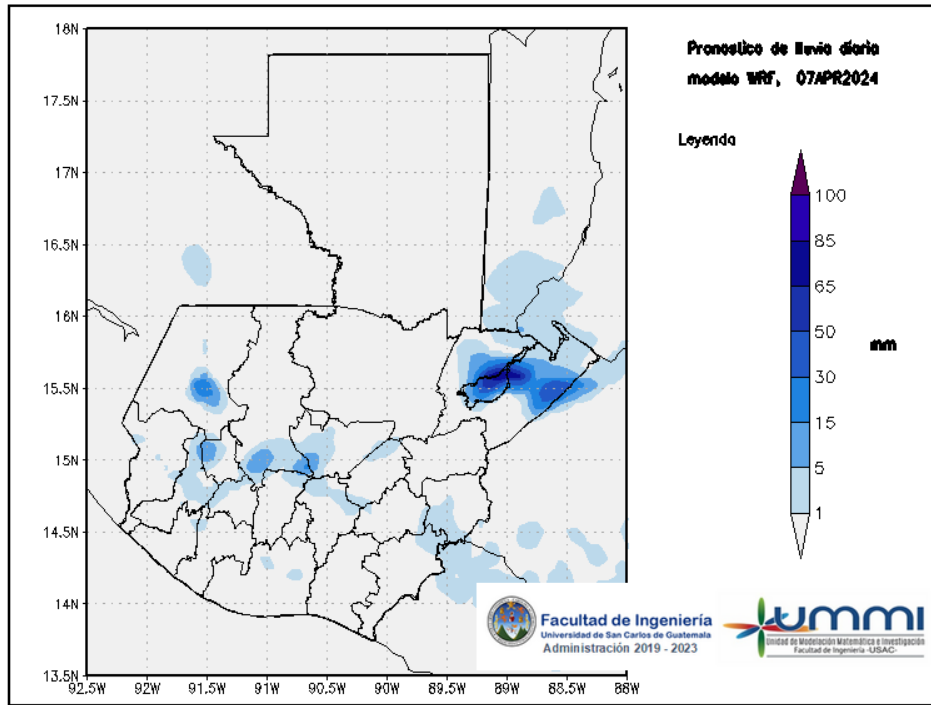
Figura 1: Pronóstico de lluvia diaria del 07 de April
