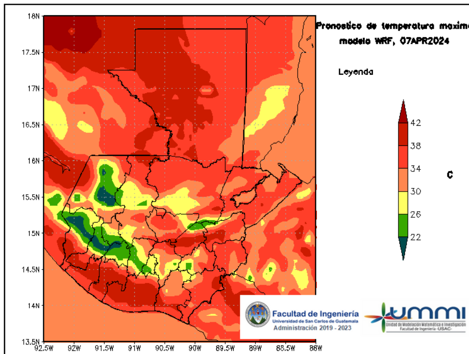
Figura 4: Pronóstico de temperatura máxima diaria del 07 de April
