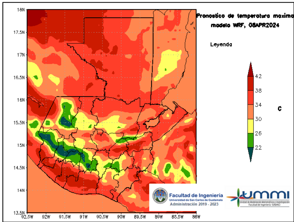
Figura 5: Pronóstico de temperatura máxima diaria del 08 de April
