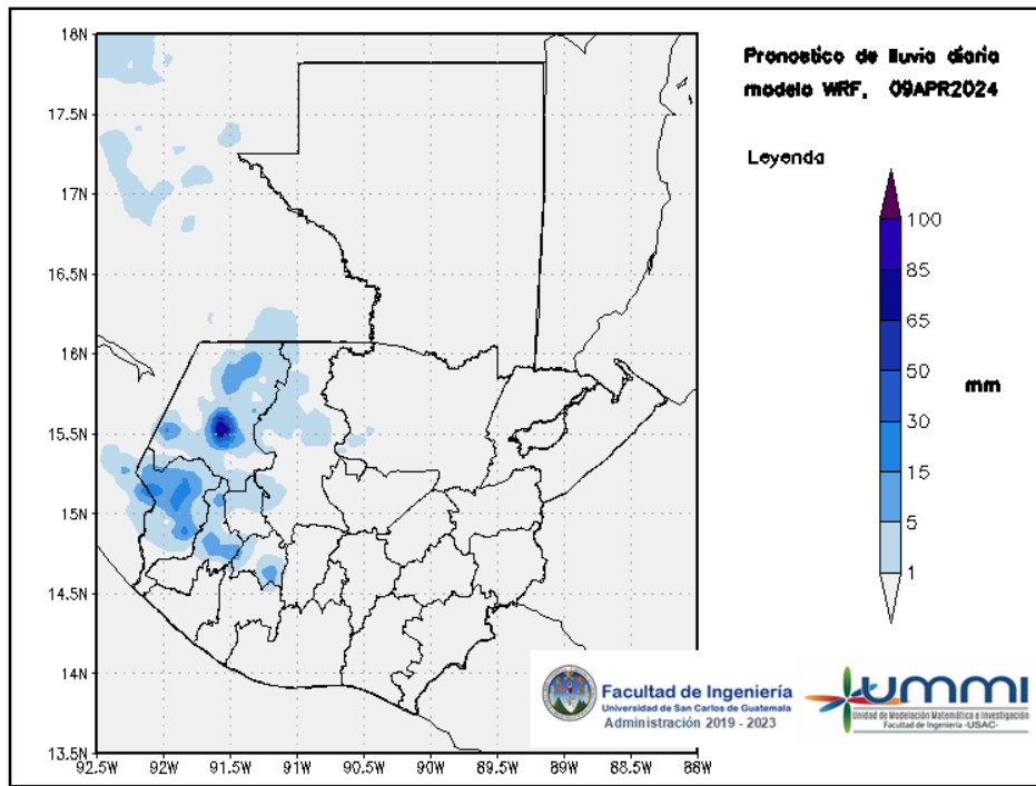
Figura 3: Pronóstico de lluvia diaria del 09 de April
