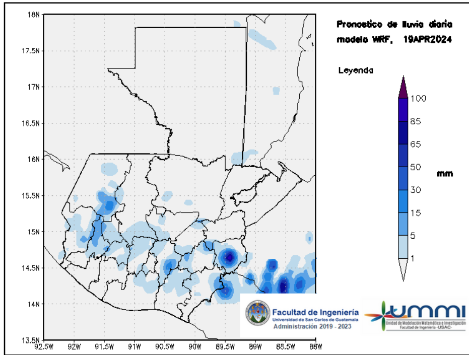
Figura 3: Pronóstico de lluvia diaria del 19 de April
