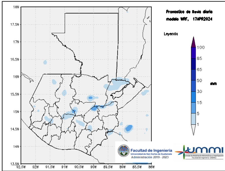
Figura 1: Pronóstico de lluvia diaria del 17 de April
