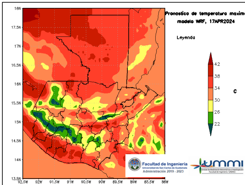
Figura 4: Pronóstico de temperatura máxima diaria del 17 de April
