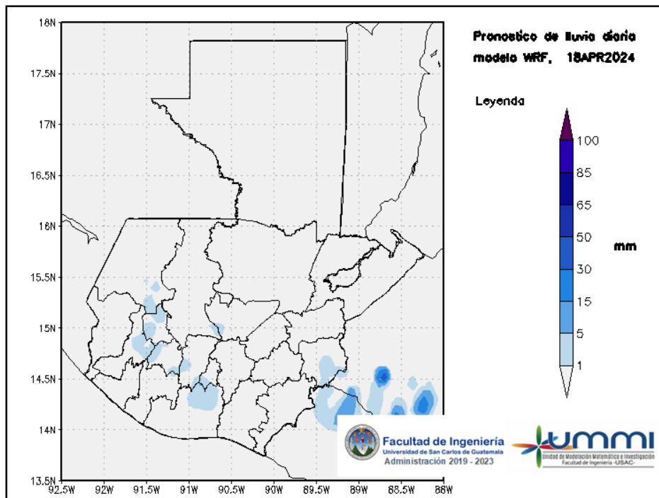
Figura 2: Pronóstico de lluvia diaria del 18 de April
