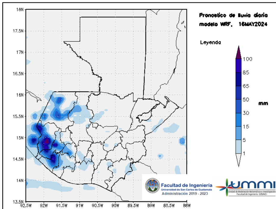
Figura 2: Pronóstico de lluvia diaria del 16 de May
