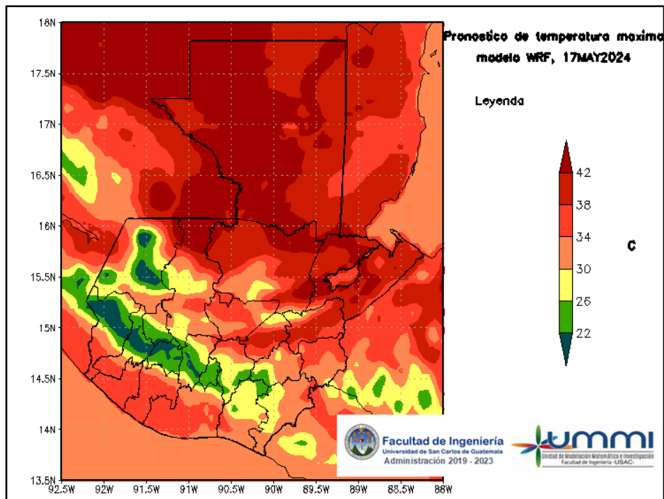
Figura 6: Pronóstico de temperatura máxima diaria del 17 de May
