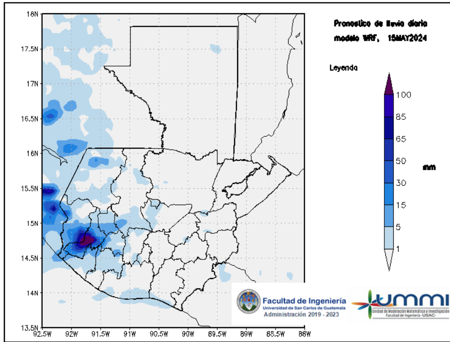
Figura 1: Pronóstico de lluvia diaria del 15 de May
