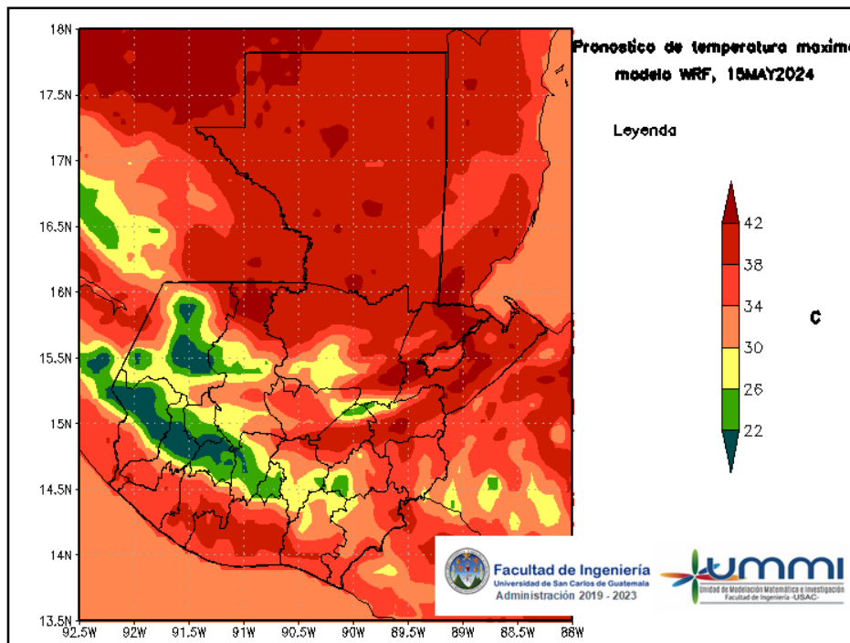
Figura 4: Pronóstico de temperatura máxima diaria del 15 de May
