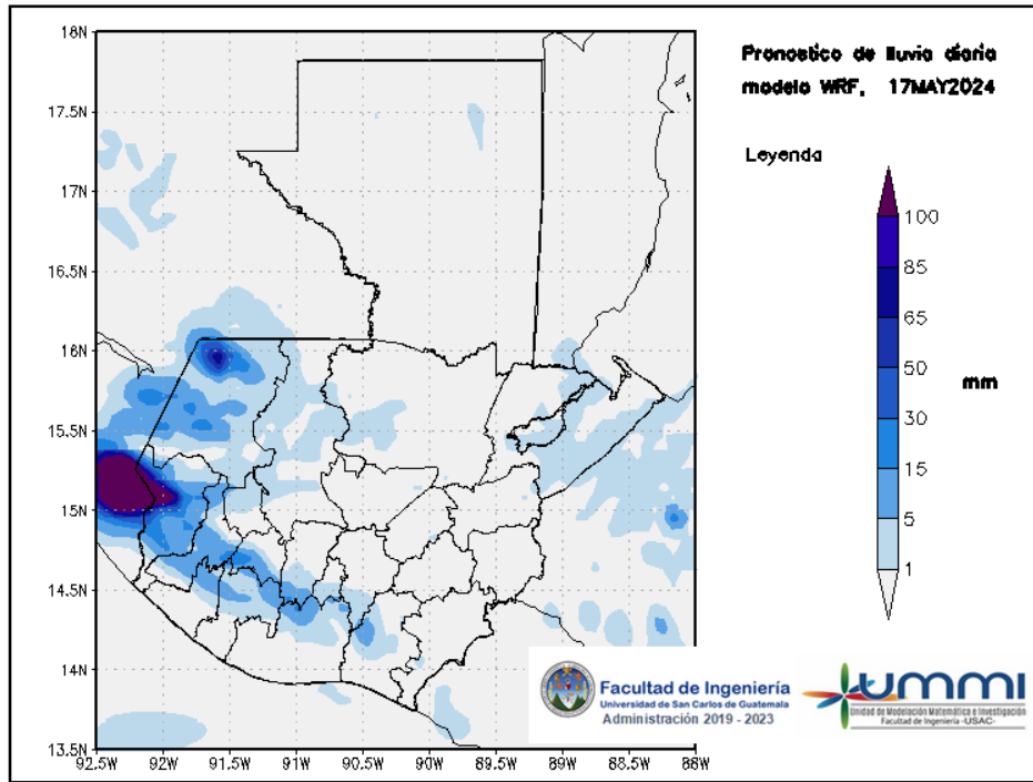
Figura 3: Pronóstico de lluvia diaria del 17 de May
