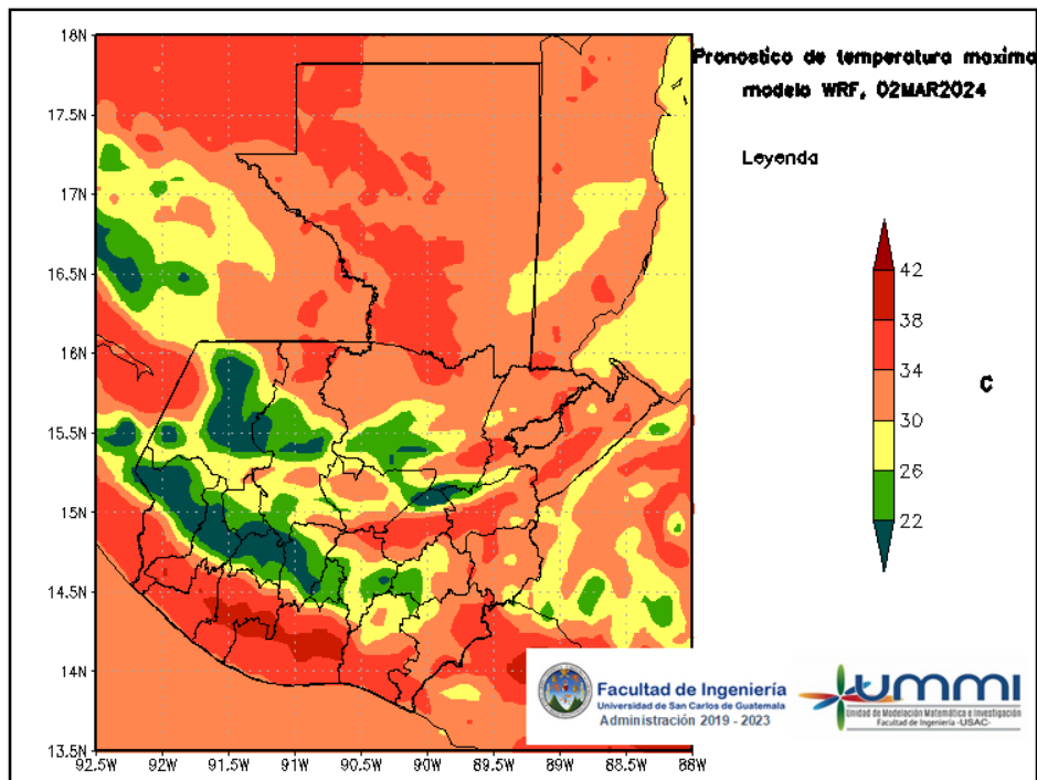
Figura 6: Pronóstico de temperatura máxima diaria del 02 de March
