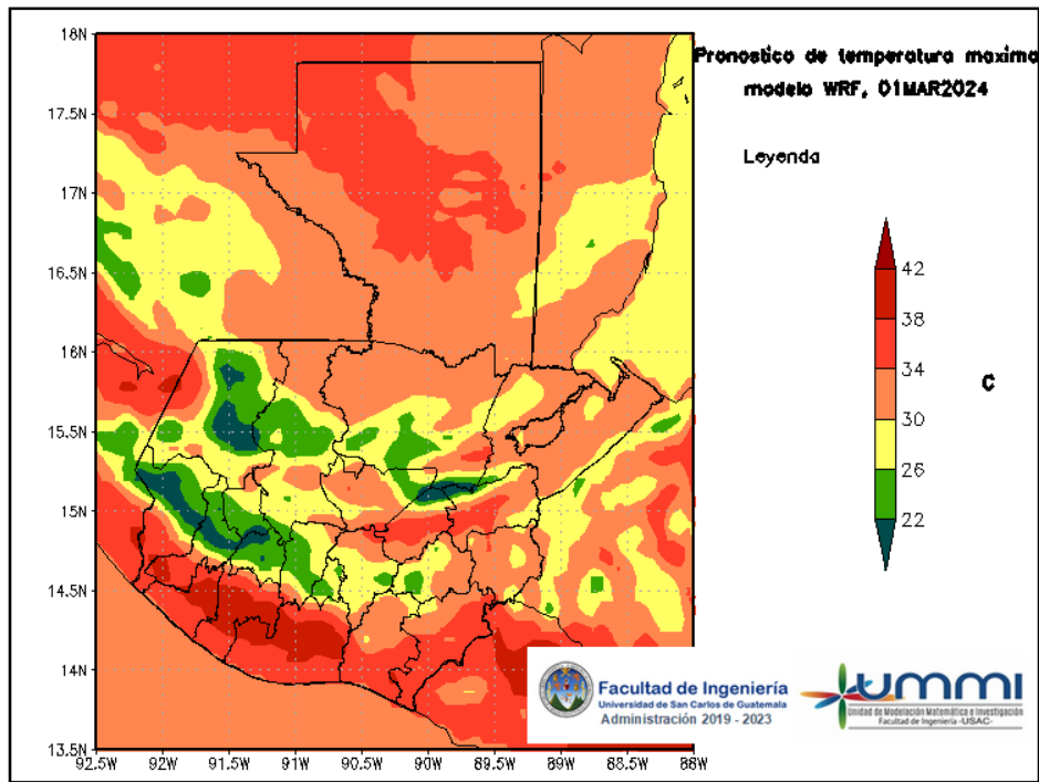
Figura 5: Pronóstico de temperatura máxima diaria del 01 de March
