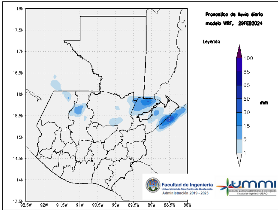
Figura 1: Pronóstico de lluvia diaria del 29 de February
