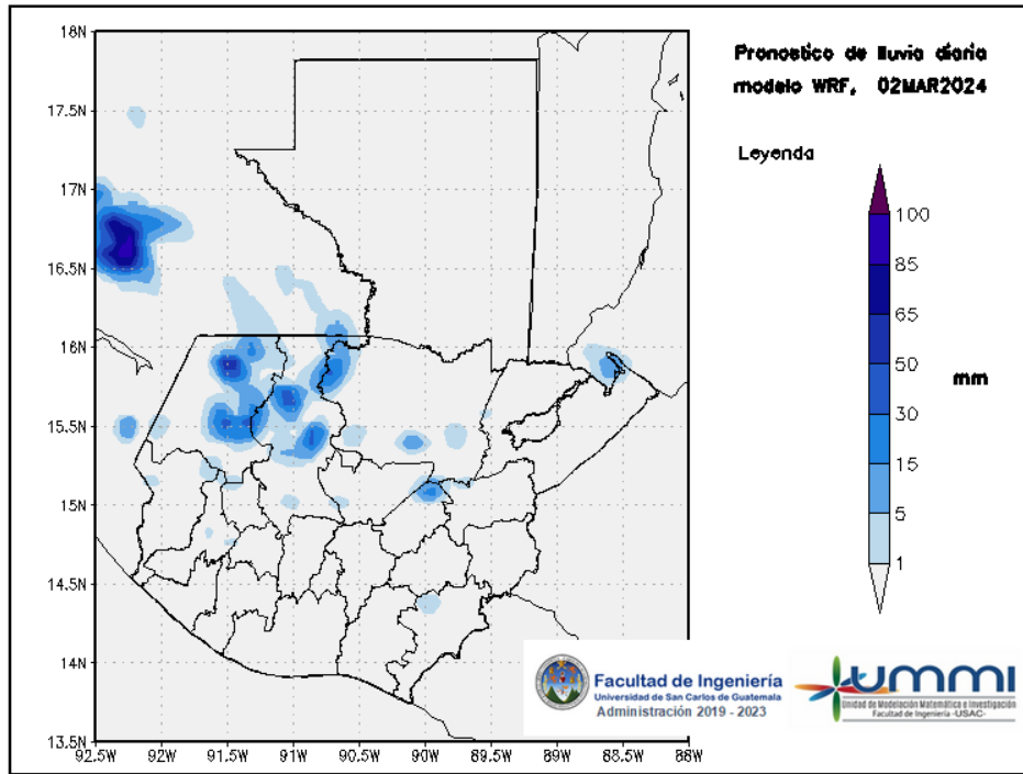
Figura 3: Pronóstico de lluvia diaria del 02 de March
