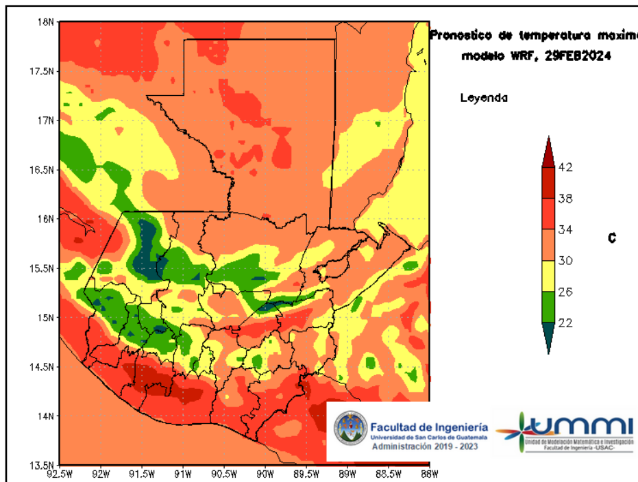
Figura 4: Pronóstico de temperatura máxima diaria del 29 de February
