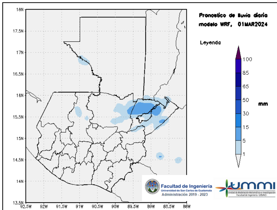
Figura 2: Pronóstico de lluvia diaria del 01 de March
