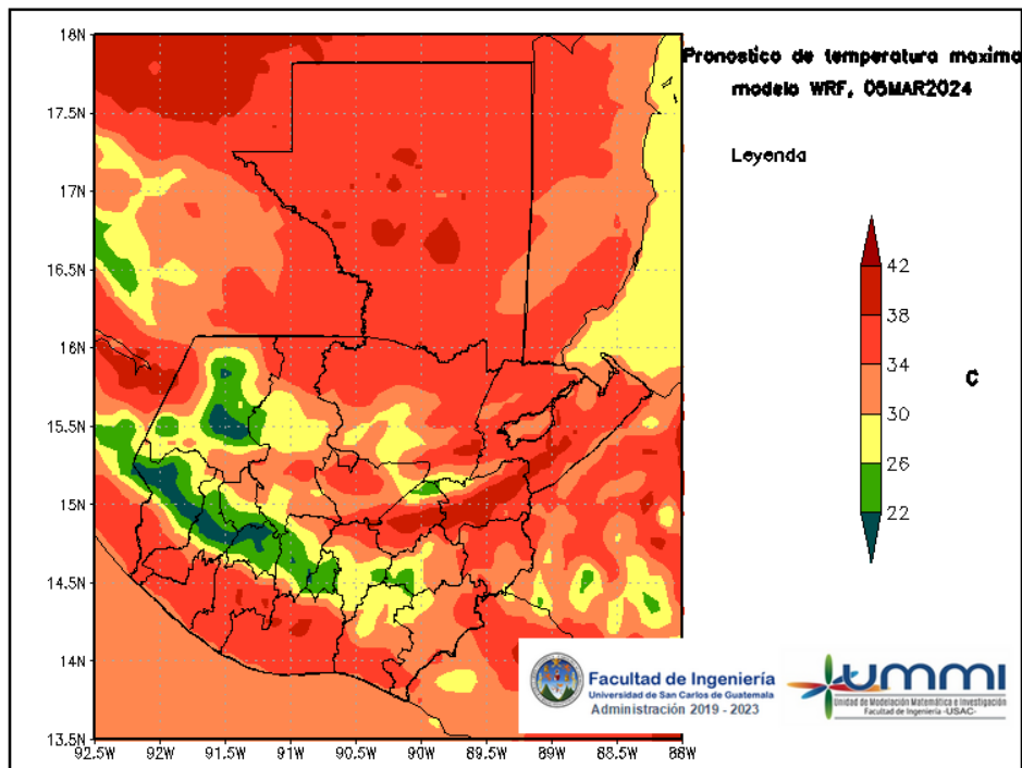
Figura 6: Pronóstico de temperatura máxima diaria del 05 de March
