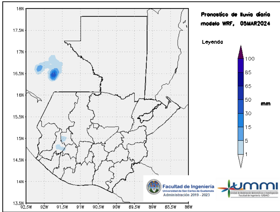
Figura 3: Pronóstico de lluvia diaria del 05 de March
