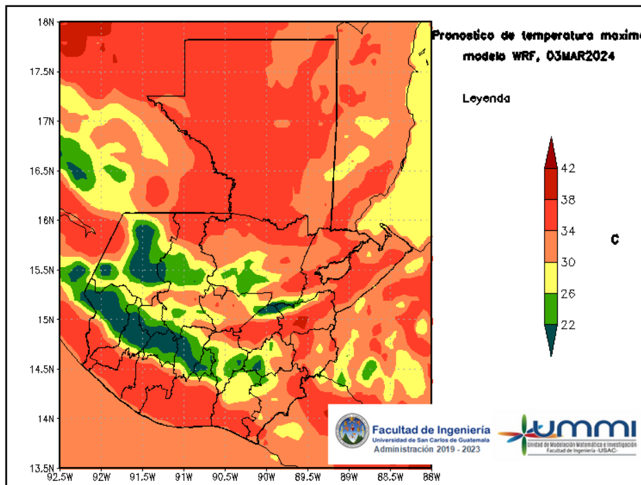
Figura 4: Pronóstico de temperatura máxima diaria del 03 de March
