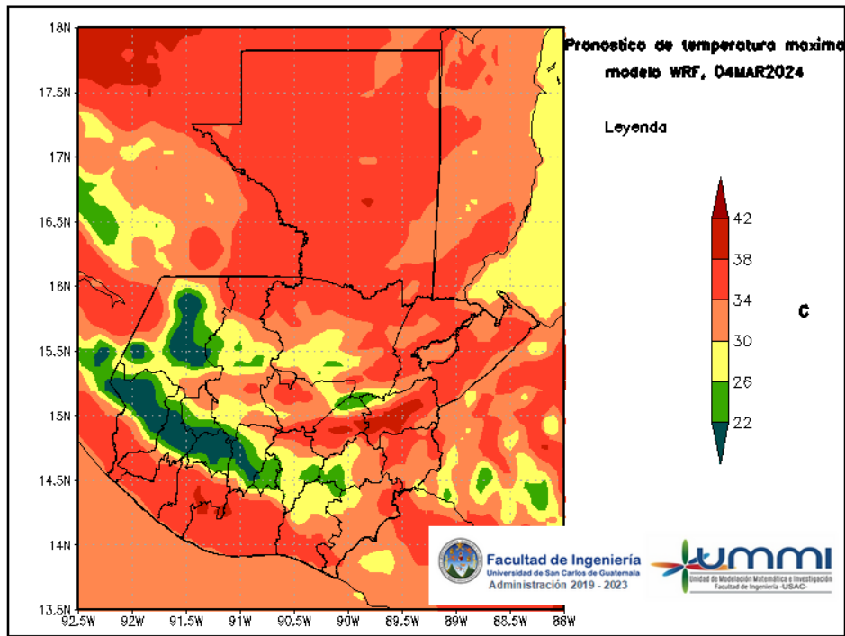
Figura 5: Pronóstico de temperatura máxima diaria del 04 de March
