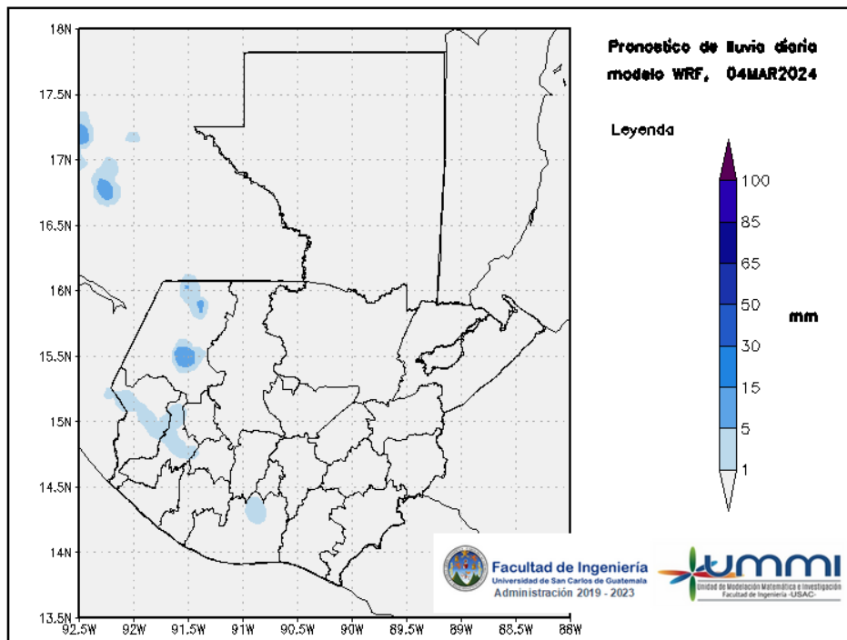
Figura 2: Pronóstico de lluvia diaria del 04 de March
