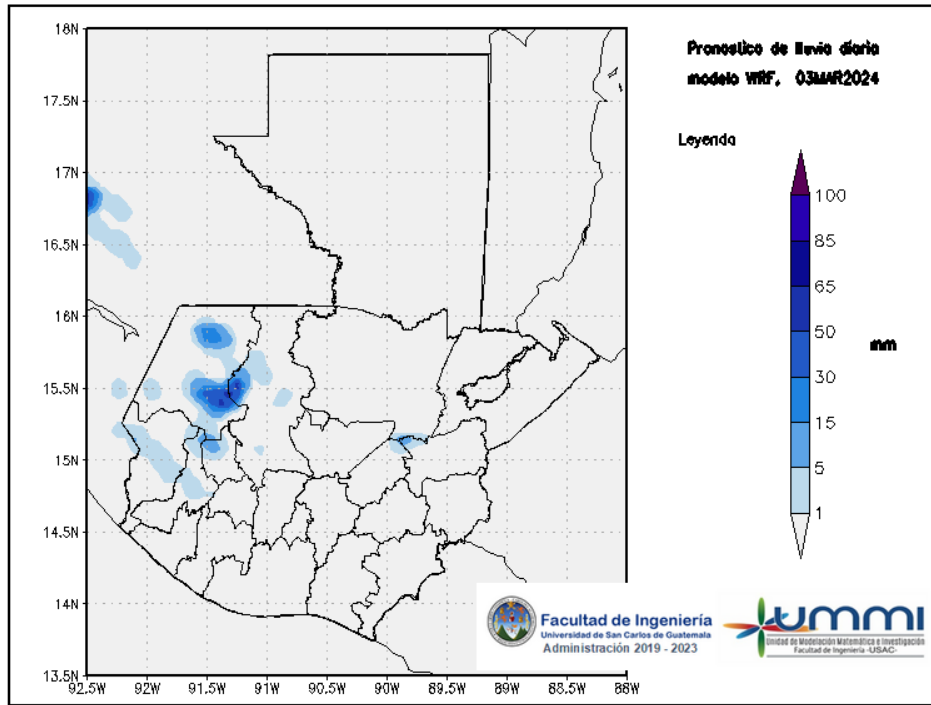
Figura 1: Pronóstico de lluvia diaria del 03 de March
